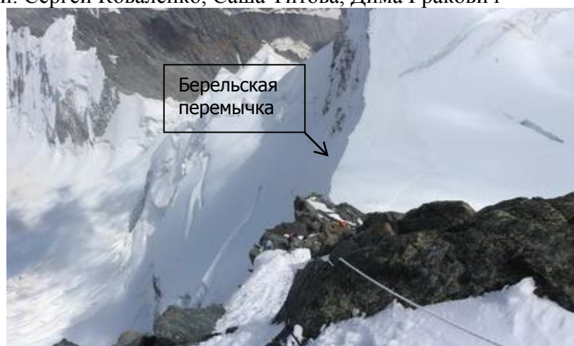
Ребро Белухи
